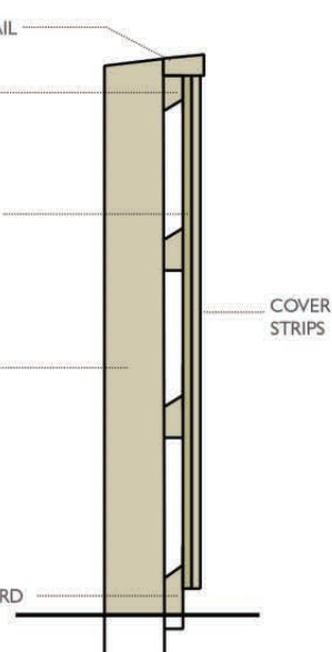
SECTION A-A
